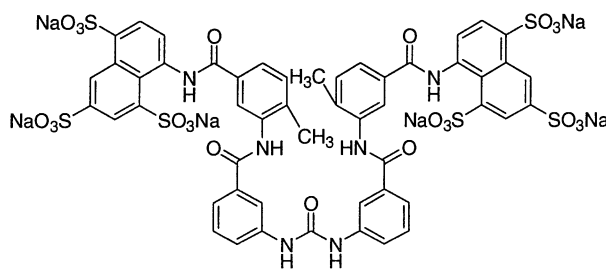
Suramin, Sodium
